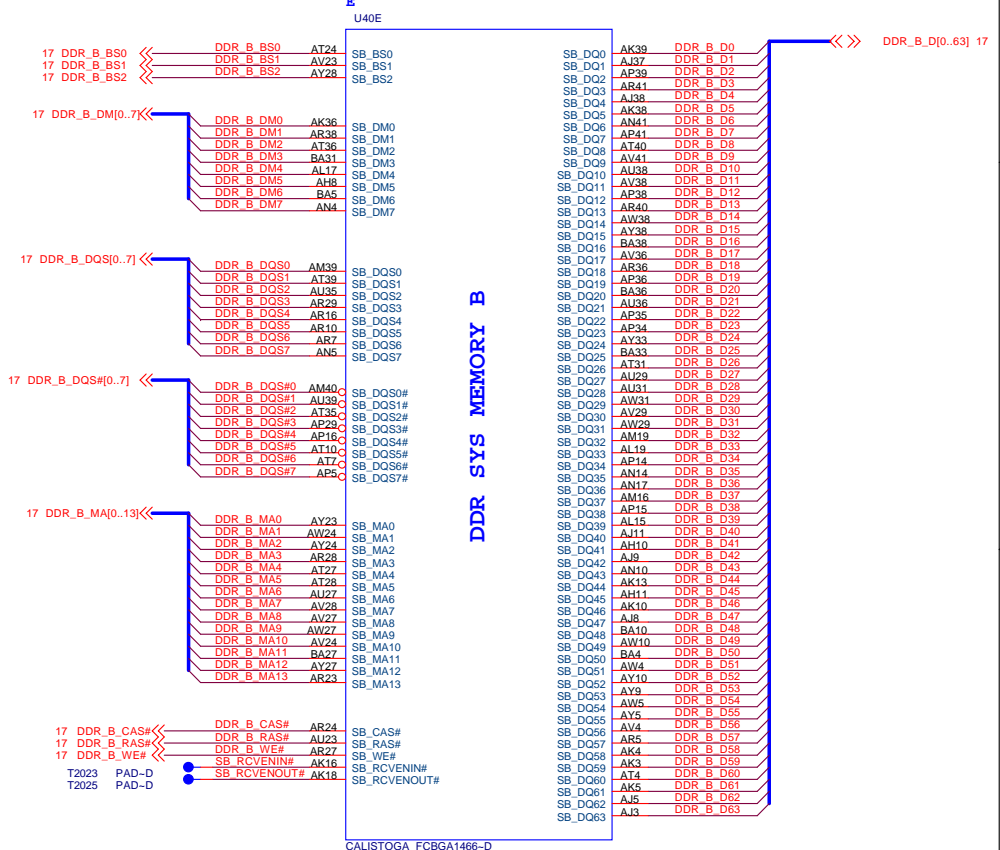
CALISTOGA_FCBGA1466-D
