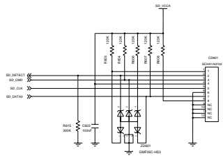
T-FLASH
