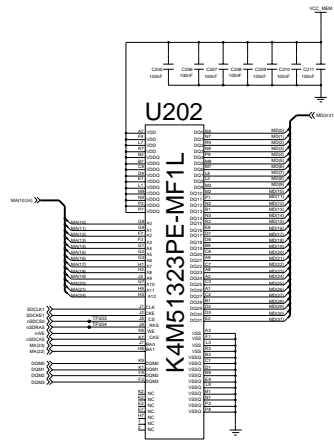
SDRAM 64MB*8 (512Mb)
