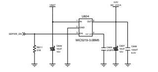
T-FLASH VOLTAGE
