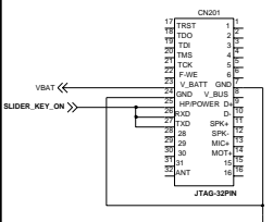
J-TAG 32 PINS
