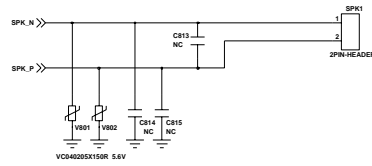
SPEAKER CON
