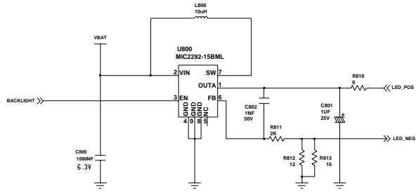
LCD BACKLIGHT IC
